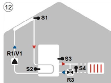
Solar mit Rücklaufanhebung
