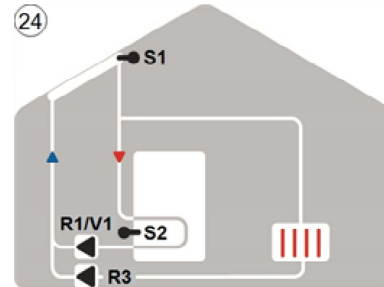
Solar mit Kühlung 2
