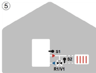
Heizkreis-Rücklaufanhebung
