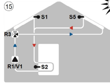
Solar mit 2 Kollektoren
