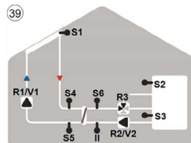
39 Solar mit Wärmetauscher, 2-Zonenspeicher und Ventil
