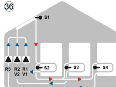
36 Solar mit 3 Speichern und 3 Pumpen
