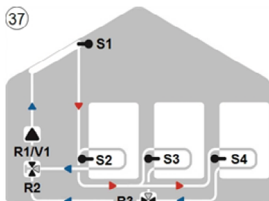
37 Solar mit 3 Speichern und 2 Ventilen
