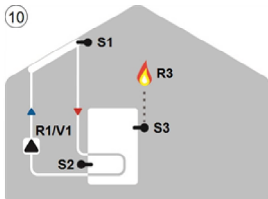
Solar mit Thermostat
