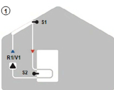
Solar mit Speicher
