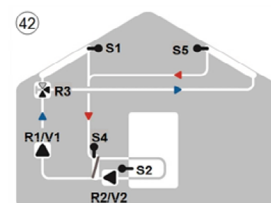
42 Solar mit 2 Kollektoren, Wärmetauscher und 2 Pumpen
