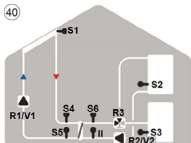
40 Solar mit Wärmetauscher, 2 Speicher und Ventil
