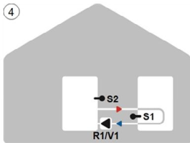
Speicherumladung
