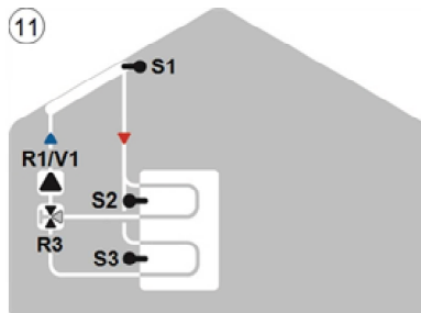
Solar mit 2 Zonenspeicher
