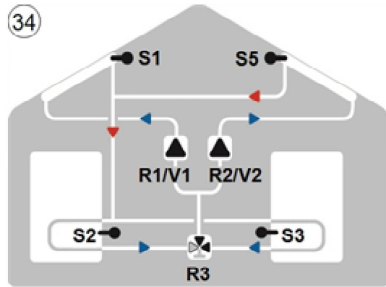
34 Solar mit 2 Kollektoren und 2 Speichern und 2 Pumpen
