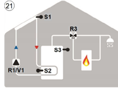
Solar mit Thermostat und Ventil
