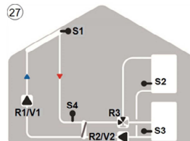
Solar mit Wärmetauscher, 2 Speichern und Ventil
