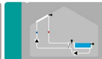
9 Solar mit Wärmetauscher (Sensor im Sekundärkreislauf) und Pool
