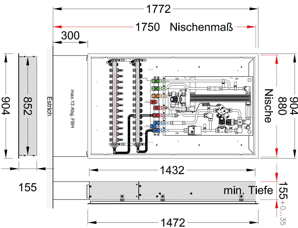
aqoloft Unterputzgehäuse "B850 x H1432"
