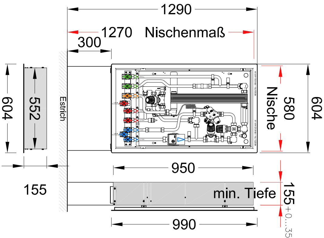
aqoloft Unterputzgehäuse "H1000 x B604"
