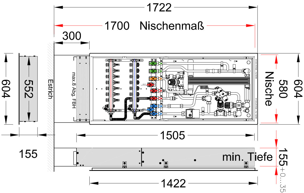
aqoloft Unterputzgehäuse "B600 x H1506"
