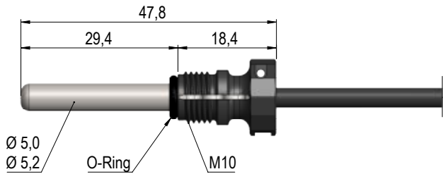
Tauchhülsentemperaturfühler mit Überwurfmutter in Verbundmaterial
