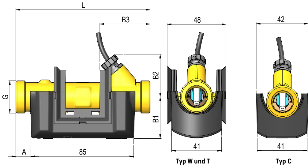
Durchflusssensor
