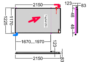
TopSol 25 - Kollektor
