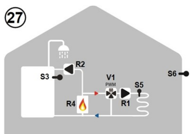
Gem. PWM-HzK, Brenner und BW Ladepumpe
