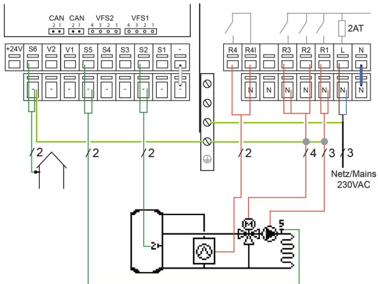
Programm 6 Gemischter HzK und WP
