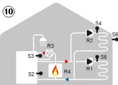
2 HzK, Kombispeicher, BW-Ventil und Brenner
