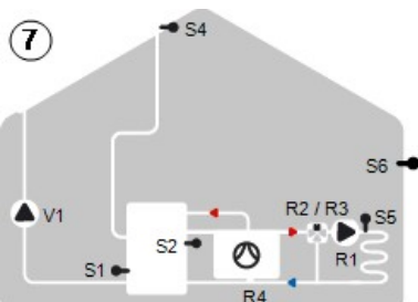
Gem. HzK, WP und Solar
