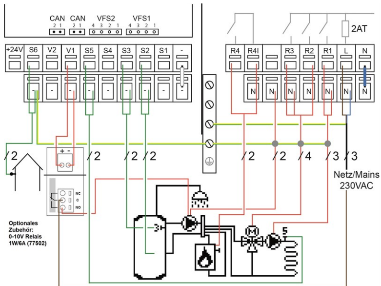
Programm 17 Gemischter HzK, Speicher und Brenner
