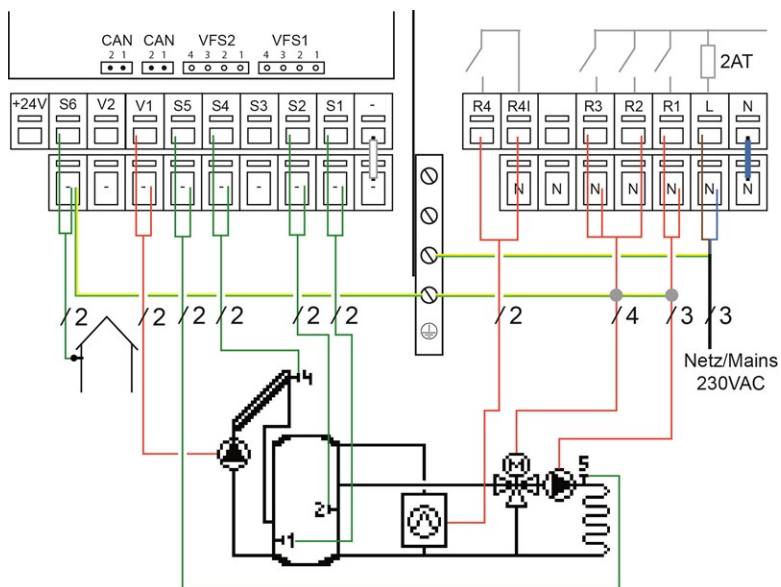
Programm 7 Gemischter HzK, WP und Solar
