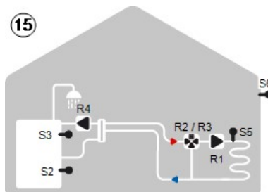
Gem. HzK und Kombispeicher
