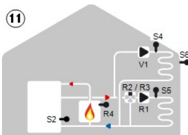
Gem. HzK, ungem. HzK und Brenner
