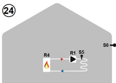
Gem. PWM-HzK, BW, Solar, Brenner und Zonenventil
