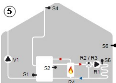
Gem. HzK, Brenner und Solar
