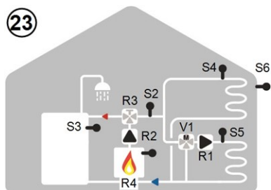
Gem. HzK mit ungem. HzK, Brenner, Direkter HzK mit Brenner
