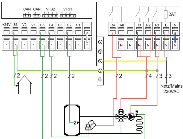
Programm 8 Gemischter HzK und Feststoffkessel
