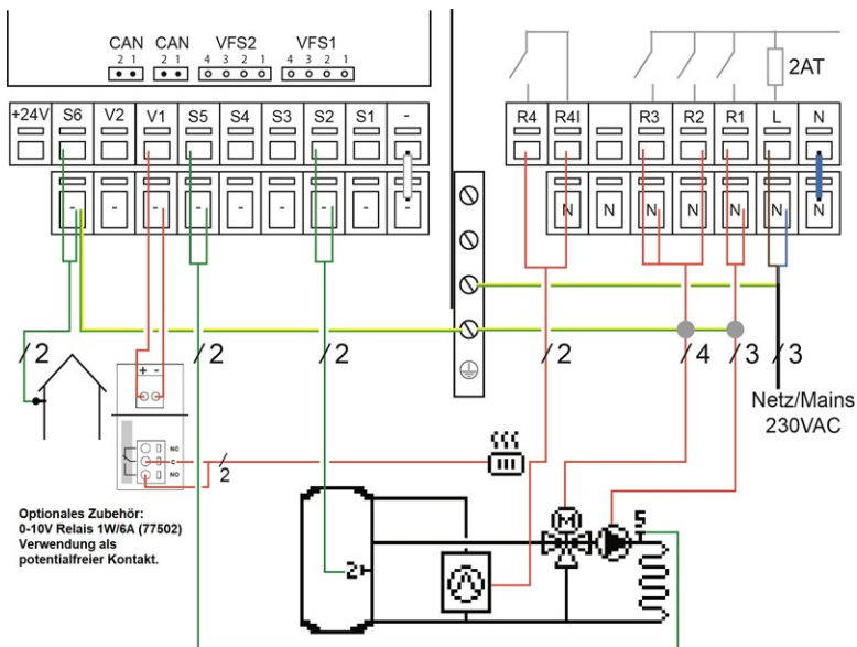
Programm 9 Gemischter HzK, WP mit Kühlfunktion
