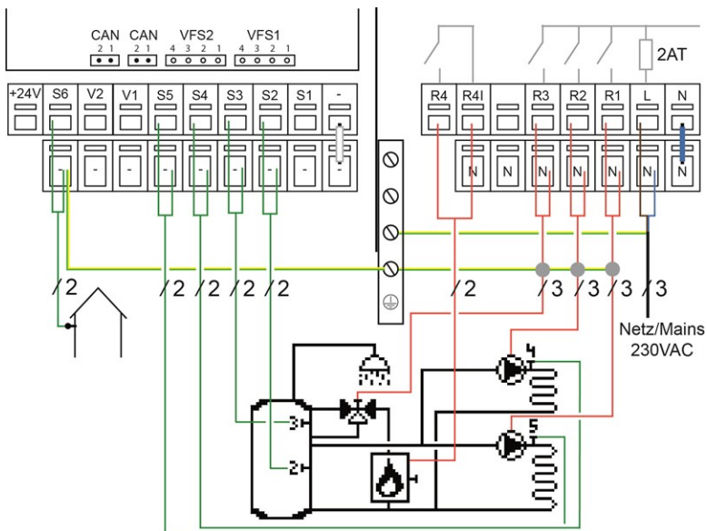
Programm 10 2 HzK, Kombispeicher, BW-Ventil und Brenner
