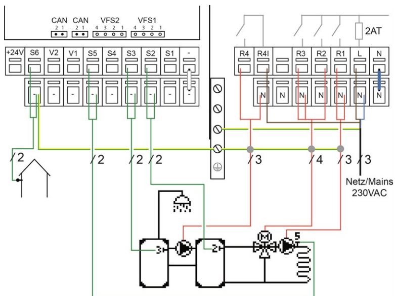
Programm 19 Gemischter HzK, BW und Speicherumladung
