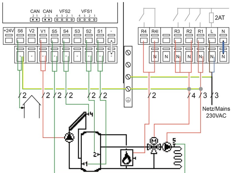
Programm 5 Gemischter HzK, Brenner und Solar
