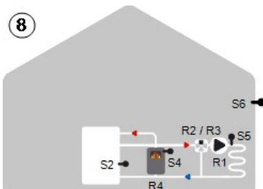
Gem. HzK und Feststoffkessel
