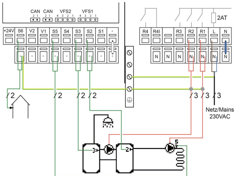
Programm 18 Ungemischter HzK, BW und Speicherumladung
