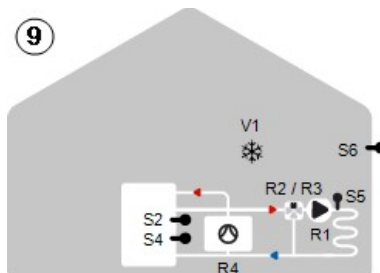
Gem. HzK, WP mit Kühlfunktion
