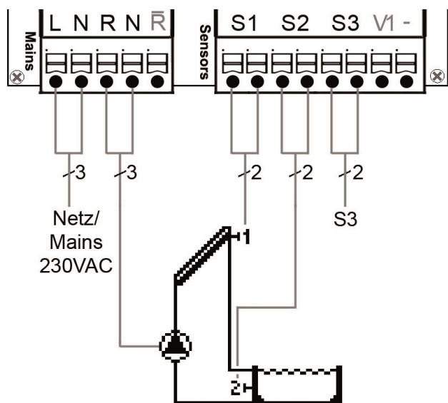
Programm 2 Solar mit Schwimmbad
