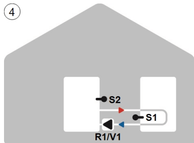
Speicherumladung
