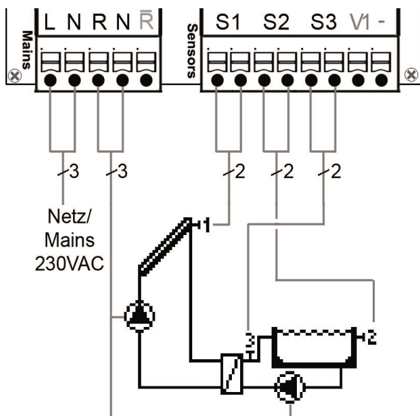
Programm 9 Solar mit Wärmetauscher und Pool
