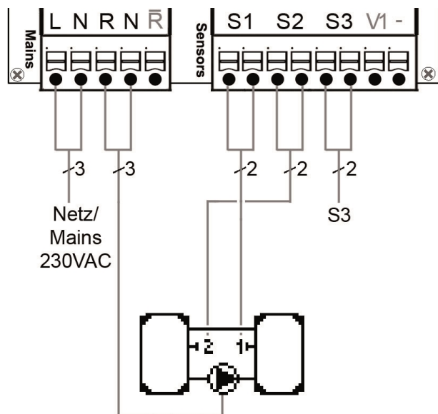
Programm 4 Speicherumladung
