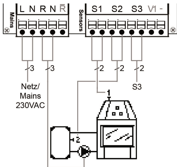
Programm 3 Feststoff mit Speicher
